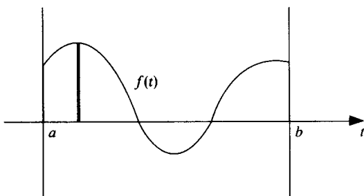
(a) \|f\|_\infty
